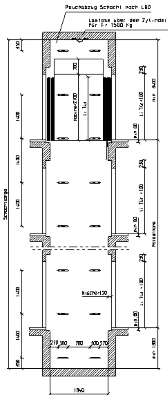
Schnitt A-A
