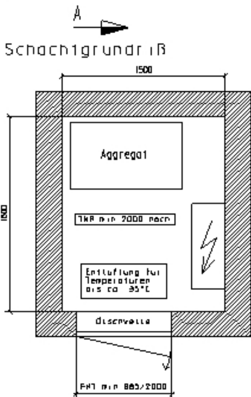
Triebwerksraumgrundriß
