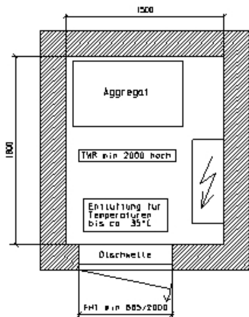
Triebwerksraumgrundiß
