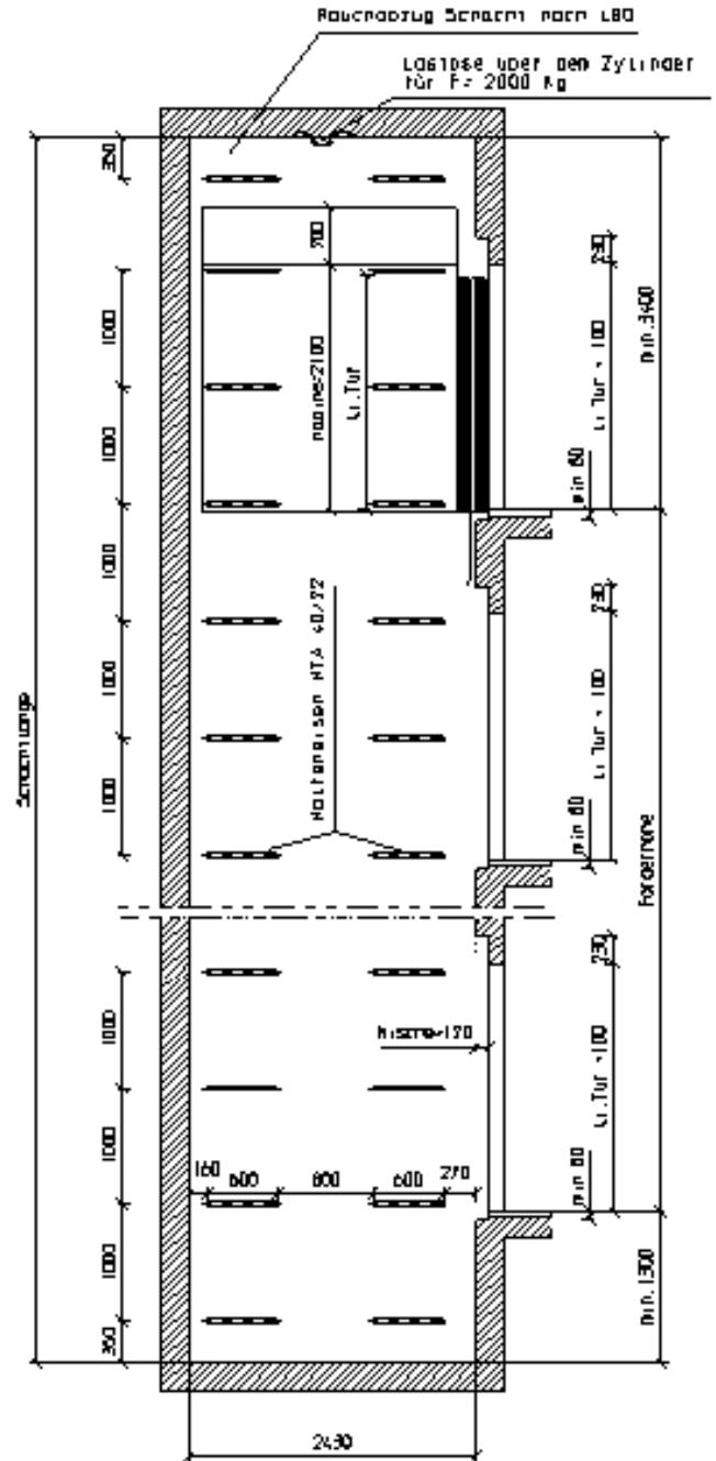
Schnitt A-A
