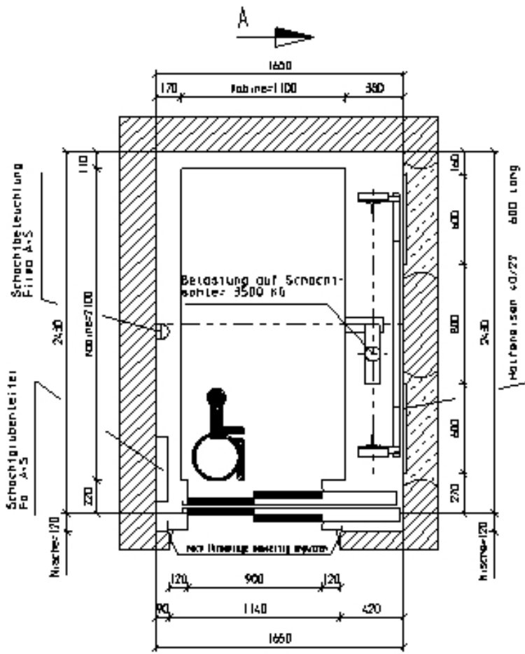
Schachtgrundiß
