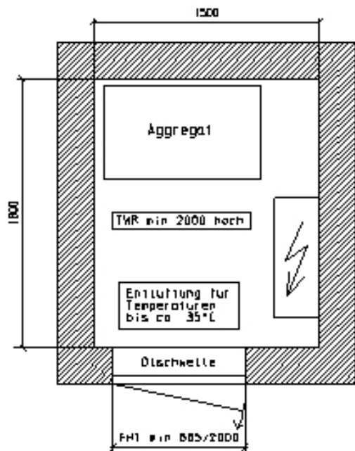
Triebwerksraumgrundiß
